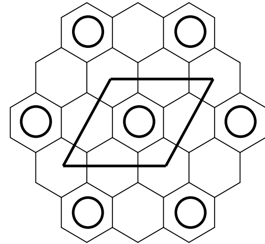
p(2x2) Superlattice
