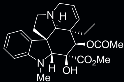
vindorosine
