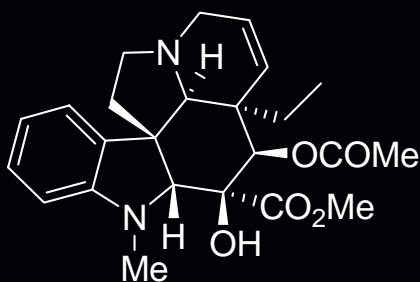
vindorosine
