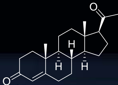
progestrone
