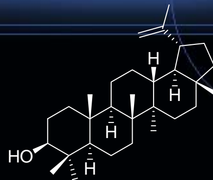
lupeol
