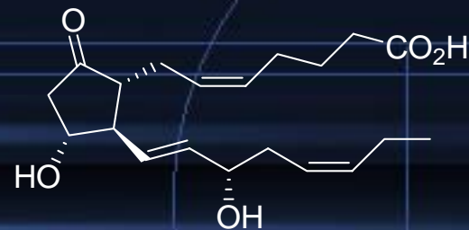
prostaglandin E 3
