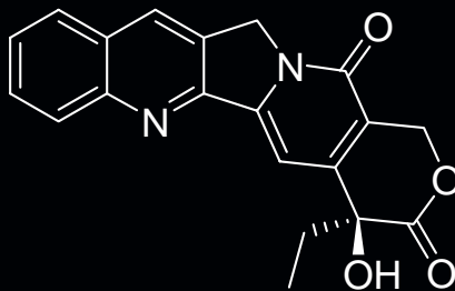
camptothecin
