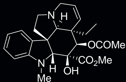
vindorosine
