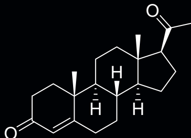
progestrone
