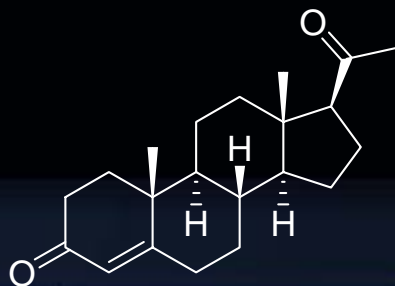
progestrone
