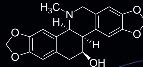
chelidone
