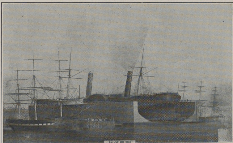
S. S. "ADRIATIC" ON BALANCE DRY DOCK.
