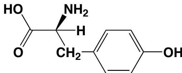
tyrosine
