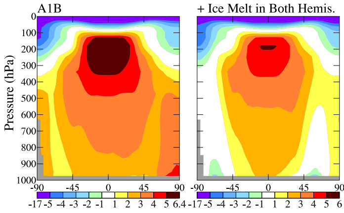
Temperature Anomaly (°C)
