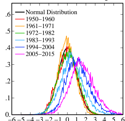
N. H. Land, Jun-Jul-Aug
