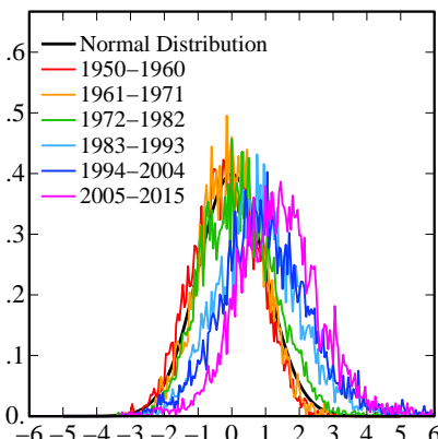
S. H. Land, Dec-Jan-Feb
