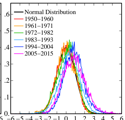
N. H. Land, Dec-Jan-Feb
