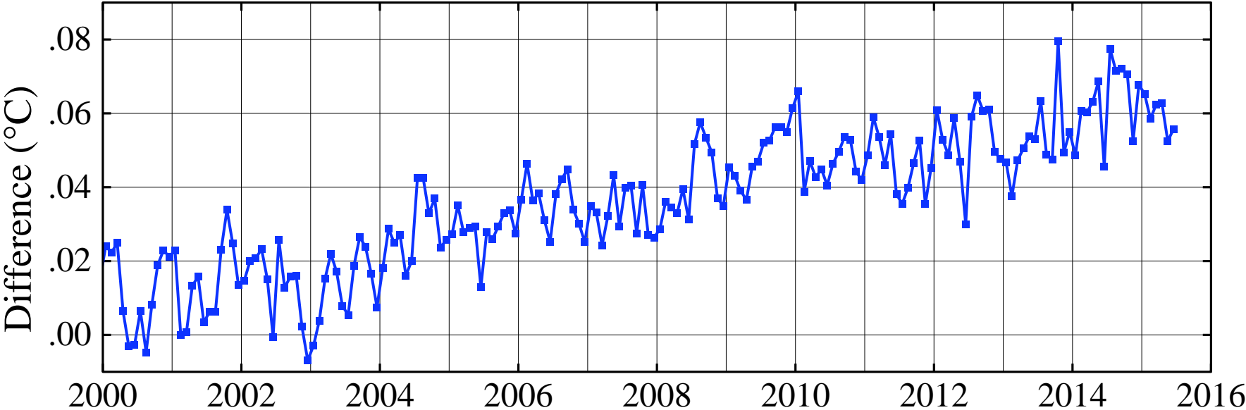
Monthly Global Surface Temperature: ERSST v4 – ERSST v3
