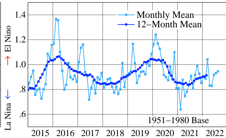
Global Mean Temperature Anomaly (°C)
