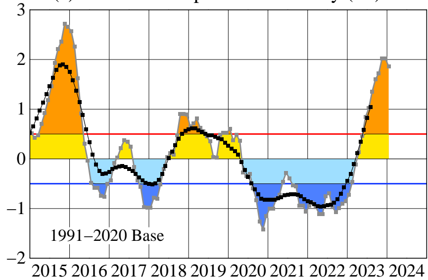
(a) Nino 3.4 Temperature Anomaly (°C)
