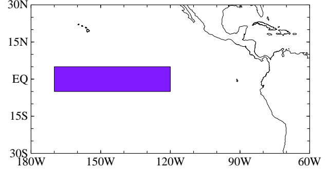
Nino 3.4
