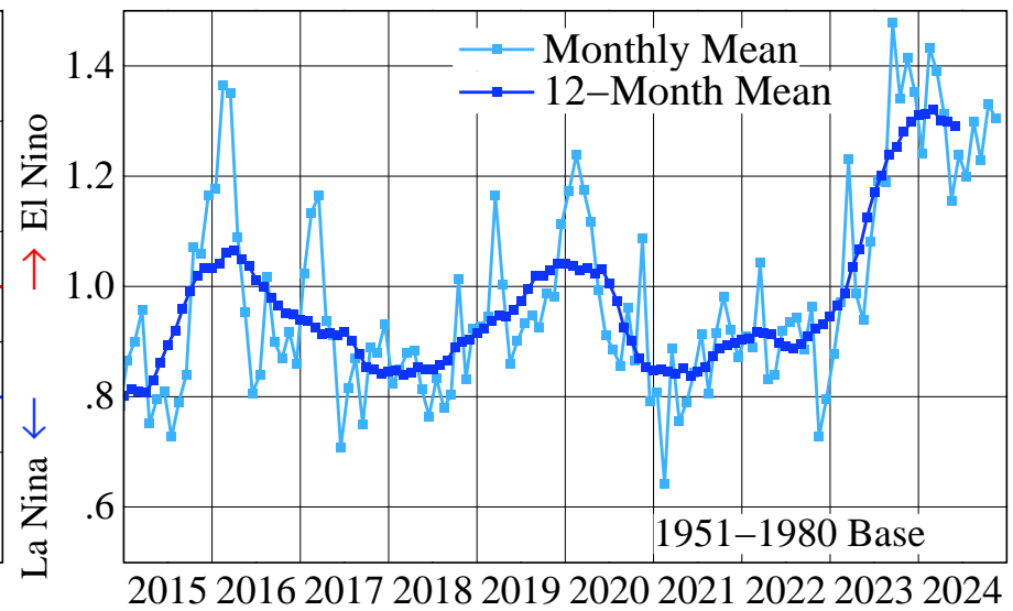
(b) Global Temperature Anomaly (°C)
