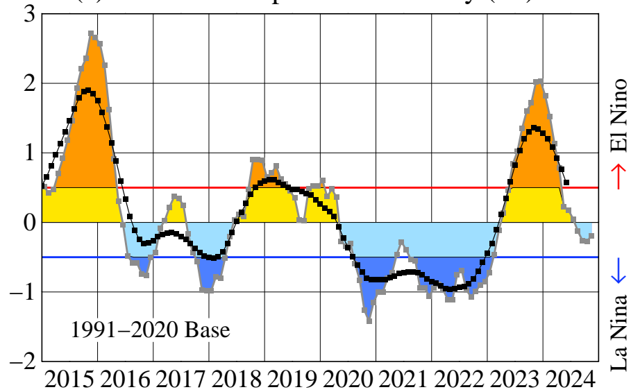
(a) Nino 3.4 Temperature Anomaly (°C)
