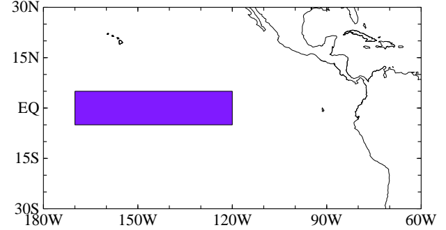
Nino 3.4
